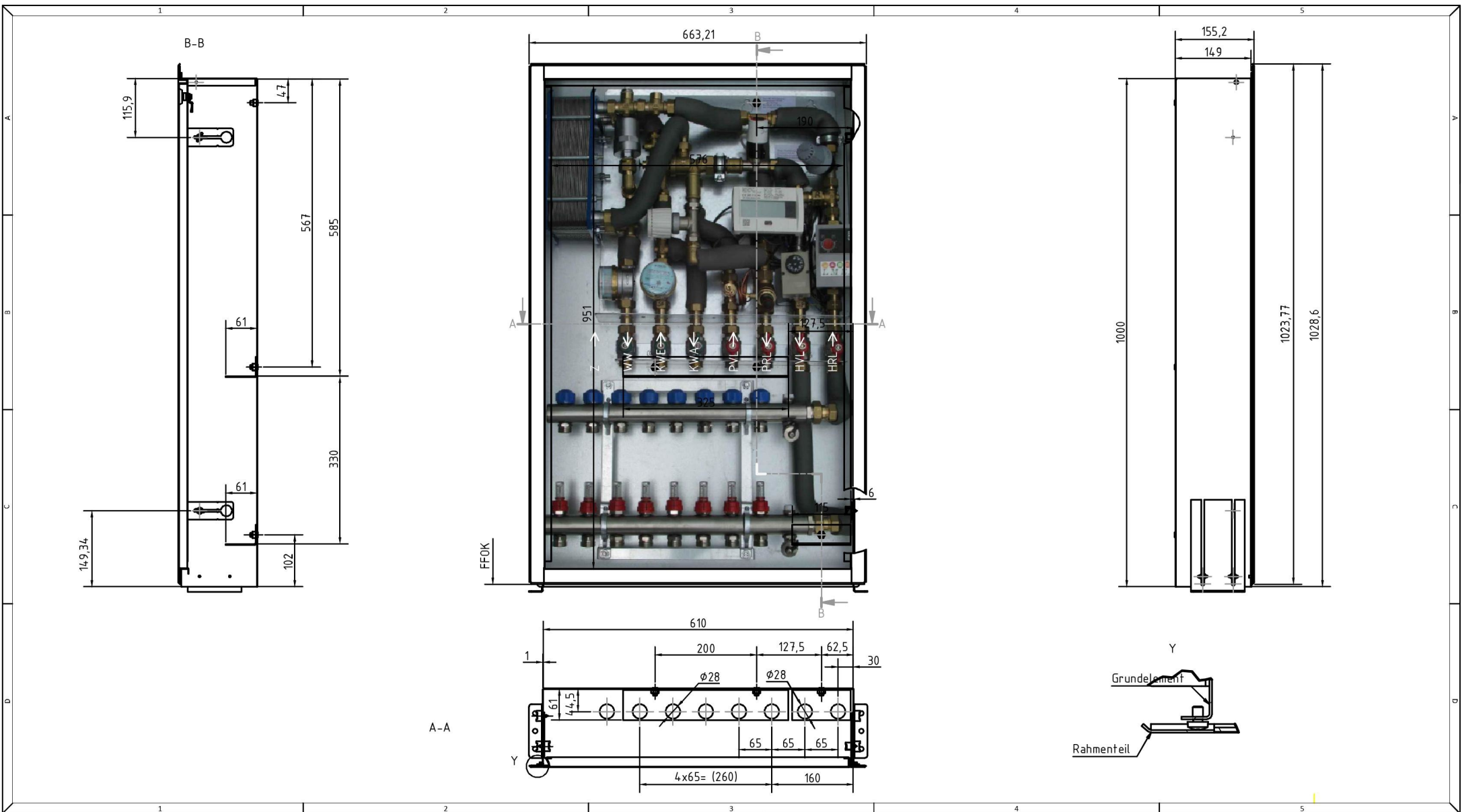
| Maßskizzen | LME-UP1000x610x150 | Wohnungsstation für FB-Heizung mit Festwertregelung, für externen FB-Verteiler 36/45/55kW
